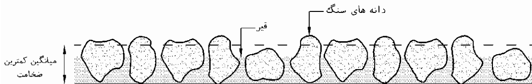
الف- موقعیت ناپایدار و نامنظم سنگدانه‌ها بلافاصله بعد از پخش روی لایه قیری راه و قبل از غلتک‌زنی.
