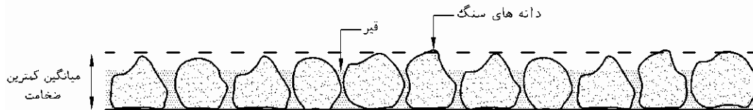
ب- موقعیت پایدار و تثبیت شده سنگدانه‌ها بعد از آمد و شد نسبتاً طولانی که روی جبهه‌های پهن و مستوی خود در لایه قیری فرو نشسته‌اند.
