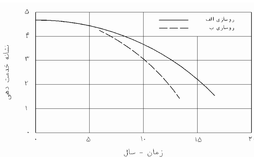
شکل ۱-۱۱- منحنی عملکرد روسازی
