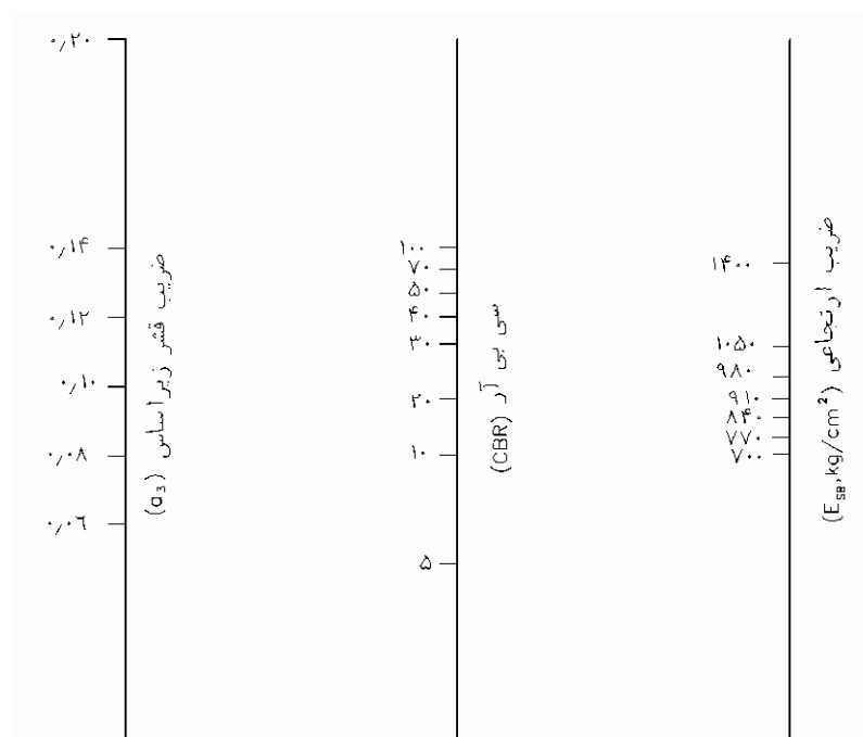
شکل ۱۱-۳- نمودار تعیین ضریب لایه زیراساس ( a_3 ) بر حسب سی‌بی‌آر و ضریب ارتجاعی
