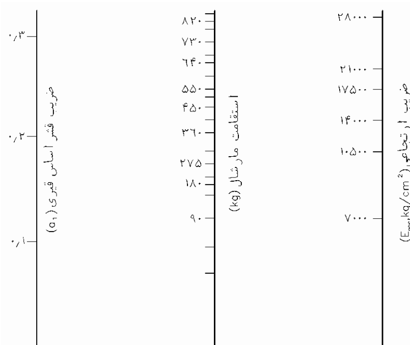
شکل ۱۱-۵- نمودار تعیین ضریب قشر اساس قیری برحسب مقاومت مارشال و ضریب ارتجاعی
