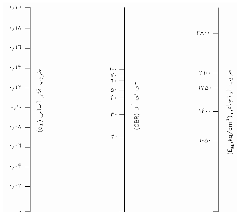
شکل ۱۱-۴- نمودار تعیین ضریب لایه اساس ( \sigma_2 ) برحسب سی بی آر و ضریب ارتجاعی
