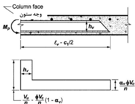
شکل ۸-۷ برش ایده‌آل در کلاhek برشی
