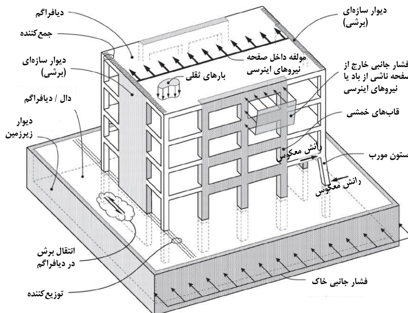
شکل ۱-۱۴ ستون‌های وارد بر دیافراگم
