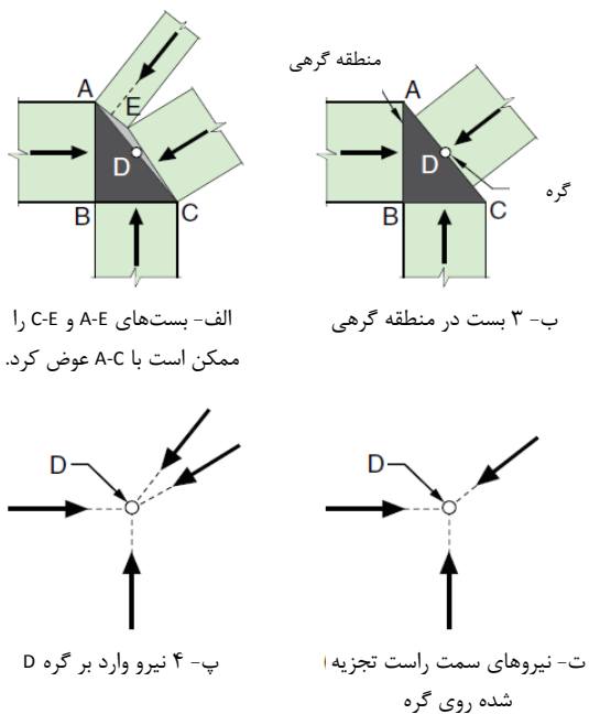
شکل ۲۲-۴ تجزیه نیروهای وارده به منطقه گرهی
