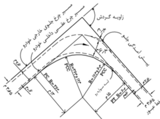
قوس مرکب سه مرکزی با شعاع‌های ۳۶ متر - ۱۲ متر - ۶۰ متر و عقب نشینی ۳۰ متر
