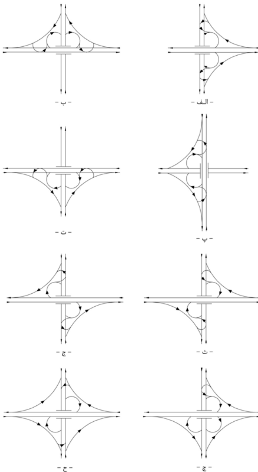
شکل ۹-۹- نمونه طرح‌های ورودی و خروجی تبادلهای نیمه‌شبه‌تبادلی
