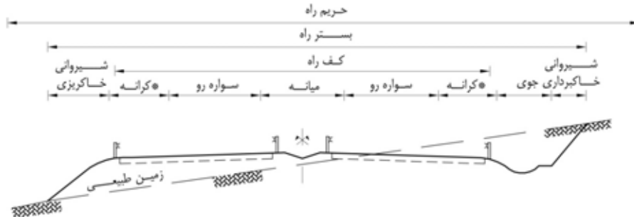
ب- جزئیات مربوط به کف راه در وضع پیوسته
