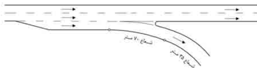
ب - قوس مرکب شعاع‌های ۳۵ متر و ۷۰ متر
