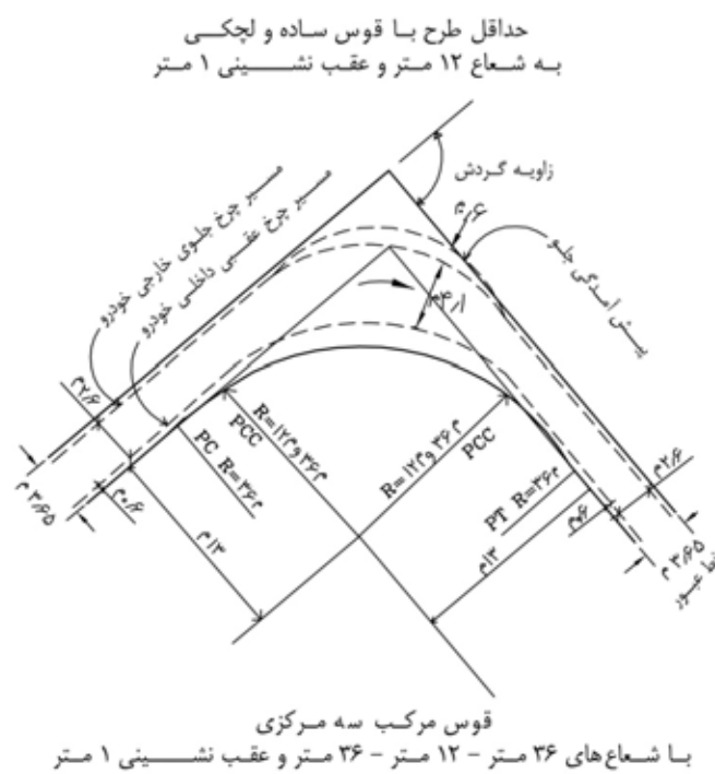
شکل ۸-۲۰- حداقل مسیر گردش برای اتوبوس نوع یک
