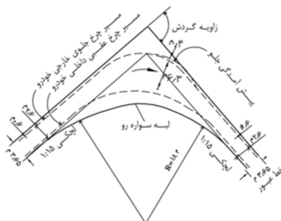
حداقل طرح با قوس ساده و لجکی به شعاع ۱۸ متر با عقب نشینی ۱ متر
