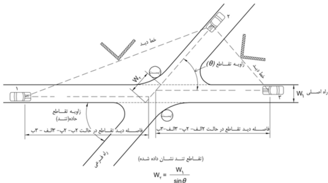
شکل ۸-۳۸- مثلث دید در تقاطع اریب
