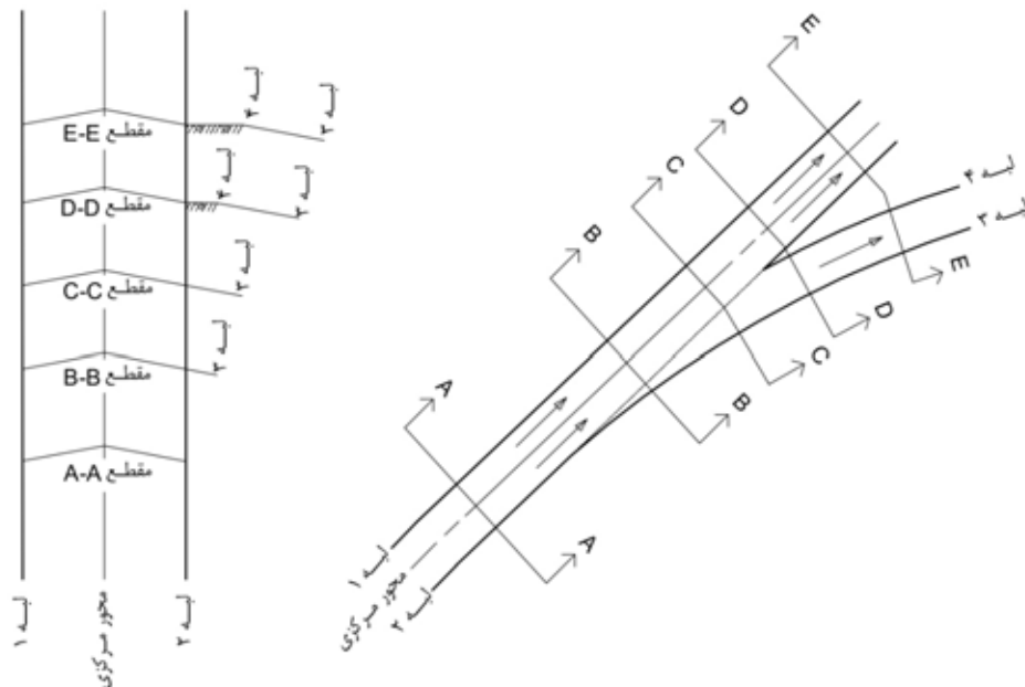
شکل ۸-۲۹- نحوه تأمین بر بلندی در پایانه- جداولگی از خط مستقیم
