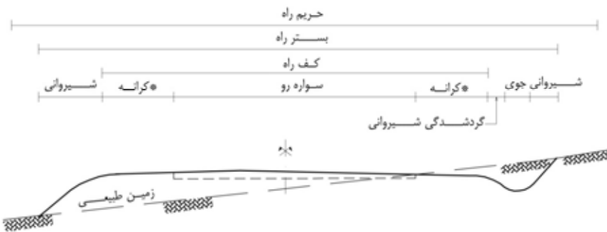
ب- جزئیات مربوط به کف راه دوخطه دو طرفه
