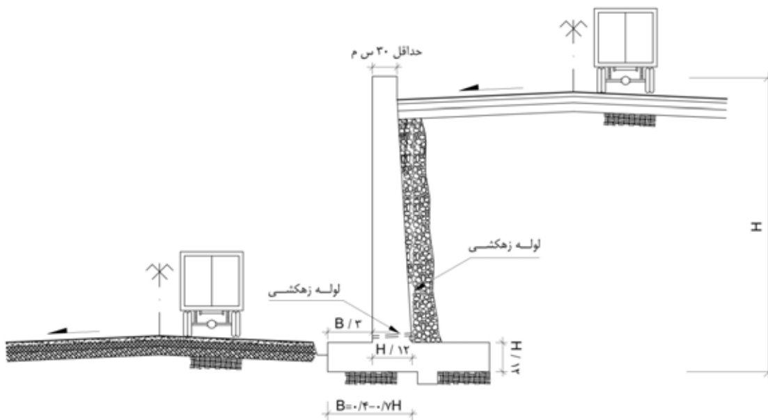
شکل ۶-۱۴ - دیوار حایل طره‌ای
