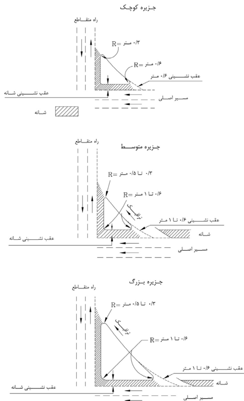
شکل ۸-۲۶- جزئیات طرح جزیره‌ها
