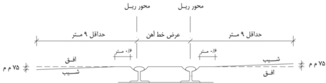
شکل ۸-۵۰- تقاطع راه-راه‌آهن
