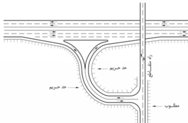
ت- محدوده کنترل دسترسی در تقاطع همسطح با راه (ملک خصوصی در داخل گردراه)
