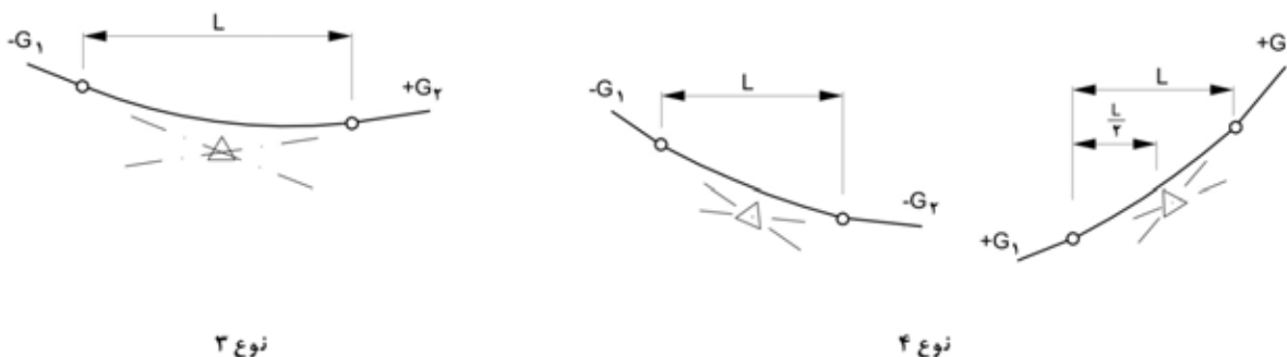
ب - انواع قوس‌های قائم کاسه‌ای (قوس‌های فرورفته)
