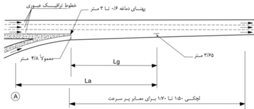
الف - طرح لجکی
