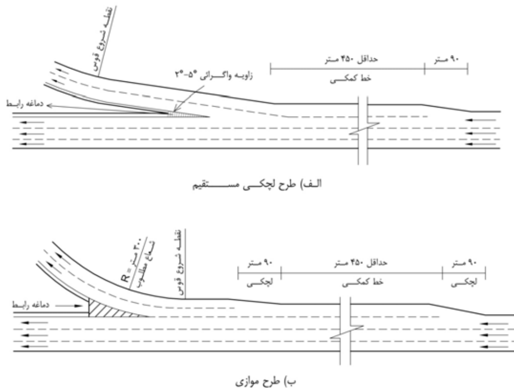
شکل ۹-۲۸- حالات‌های متداول رابط خروجی دو خطه
