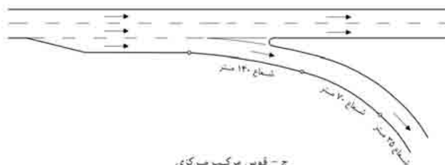
ج - قوس مرکب مرکب با شعاع‌های ۳۵ متر - ۷۰ متر و ۱۴۰ متر
