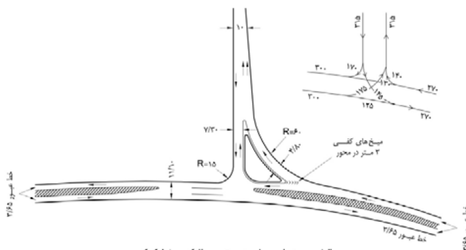
الف - سه راهی یا جزیره ترافیکی و خط کمکی (تعریف شده در محل تقاطع)
