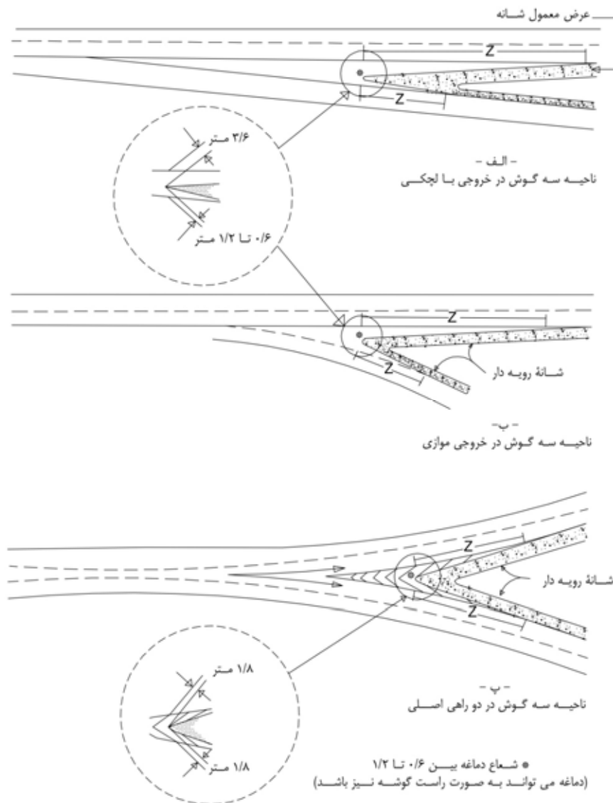
شکل ۹-۲۲- طرح‌های ناحیه سه گوش برای حالت‌های مختلف
