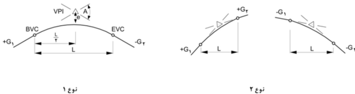
الف - انواع قوس‌های قائم گنبدی (قوس‌های برآمده)
