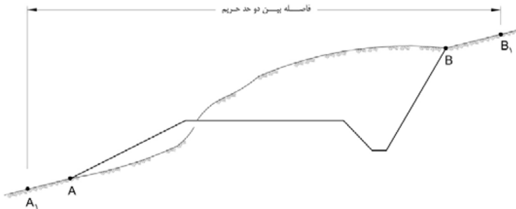
شکل ۵-۶- حریم راه
