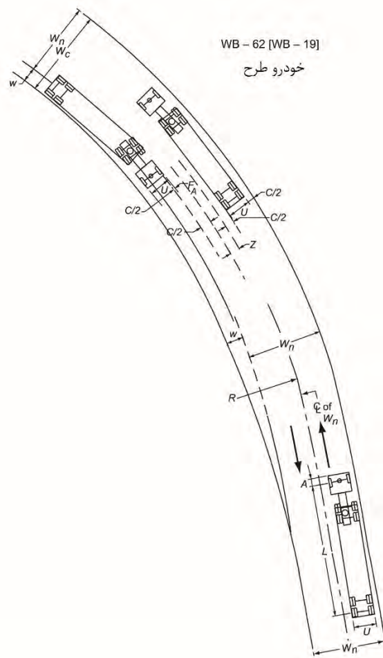
شکل ۵-۴- تعریض راه در قوس افقی
