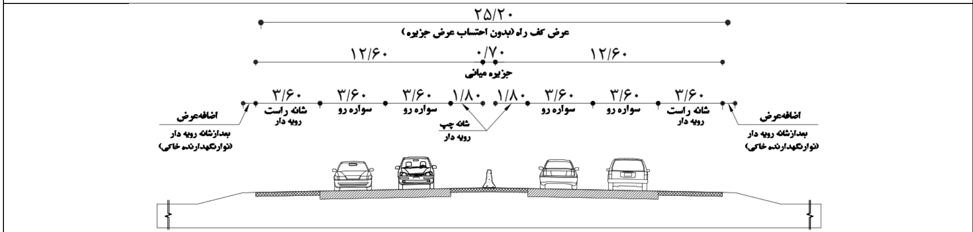
F2- آزادراه چهار خطه با DDHV برابر و بیشتر از ۲۵۰
