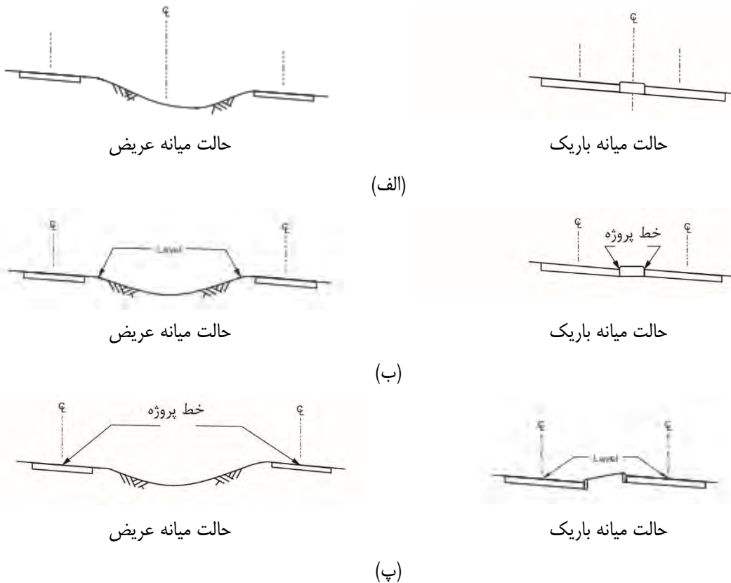
شکل ۵-۳- دوران بریلندی حول لبه خارجی در سواره روی با شیب عرضی یک طرفه
