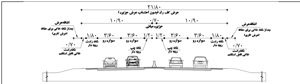
A1- راه شریانی جداشده چهار خطه
