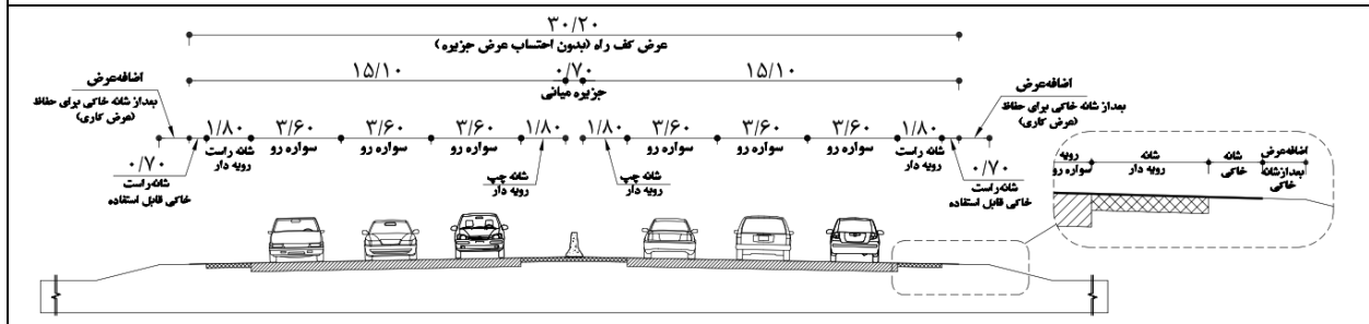
A2- راه شریانی جداشده شش خطه
