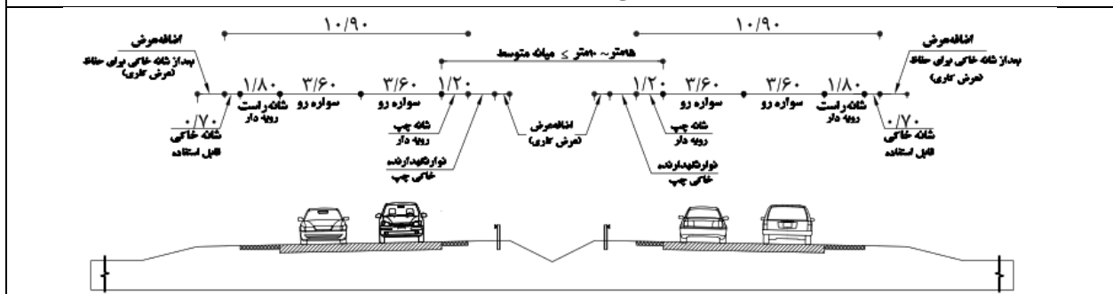
A5- راه شریانی جداشده چهار خطه با میانه متوسط
