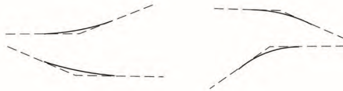
گردشگي گوشه های سواره رو در محل اعمال بریلندی
