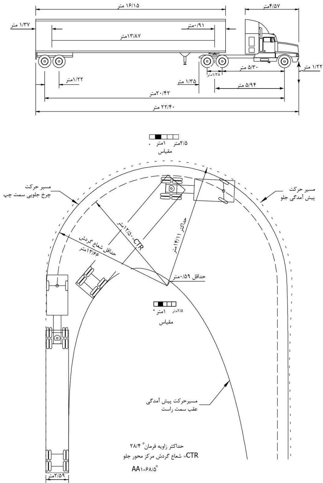
شکل ۴-۹- حدافل مسیر گردش برای وسیله طرح تریلی نوع ۳
