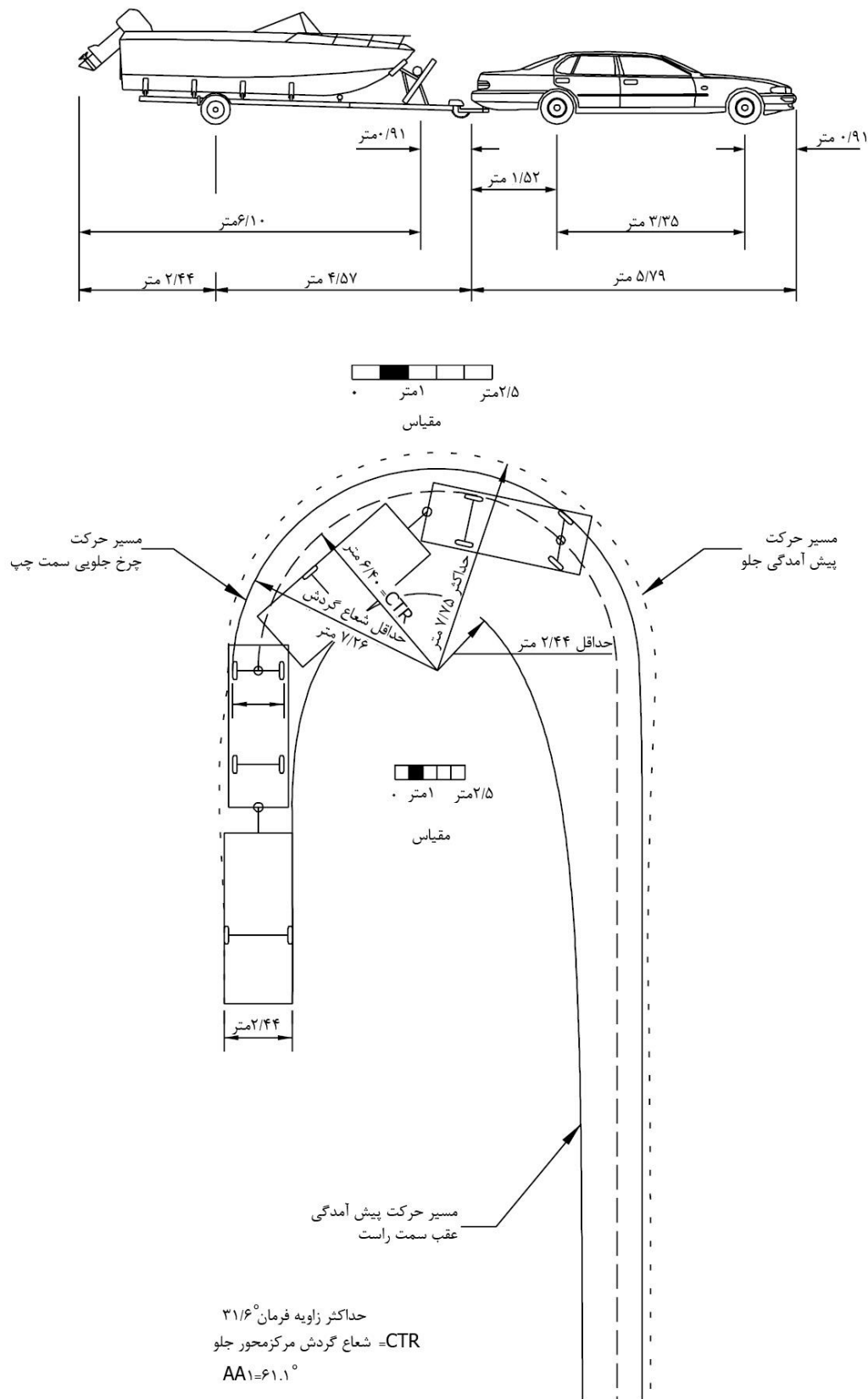
شکل ۴-۱- حداقل مسیر گردش برای وسیله طرح سواری با یدک قایق
