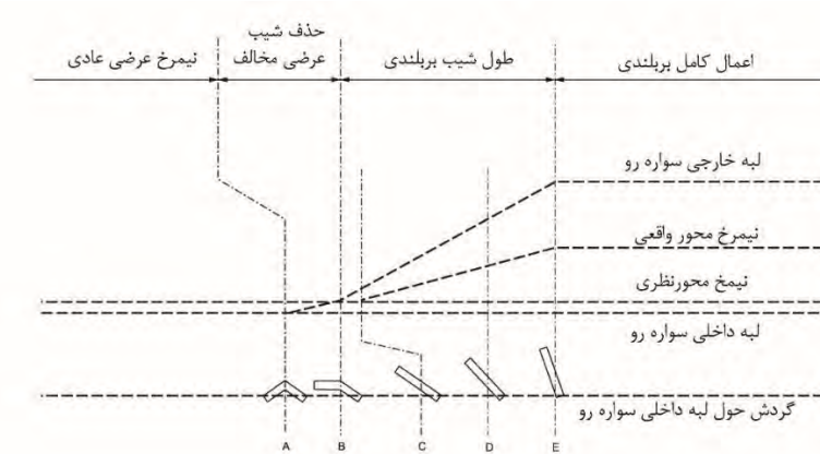
سواره رو با نیمرخ عادی حول لبه داخلی گردش می کند.
