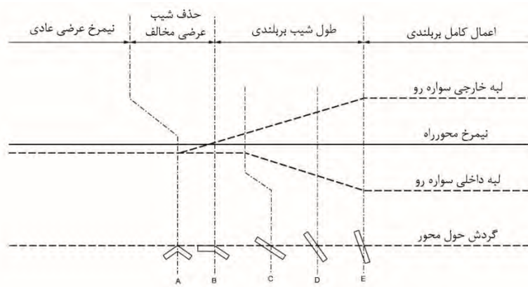
سواره رو با نیمرخ عادی حول خط محور راه گردش می کند.
