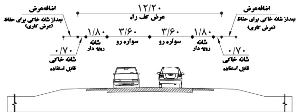
A۴- راه شریانی دو خطه با ADT بیشتر از ۲۵۰
