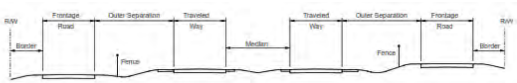
شکل ۶-۱۶- نمونه ای از مقطع عرضی راه شریانی جدا شده با احتساب راه های جانبی
