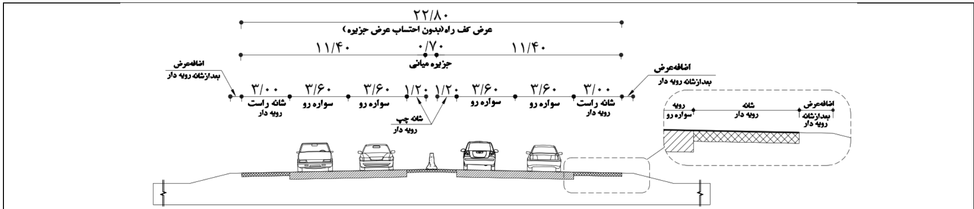
F1- آزادراه چهار خطه با DDHV کمتر از ۲۵۰
