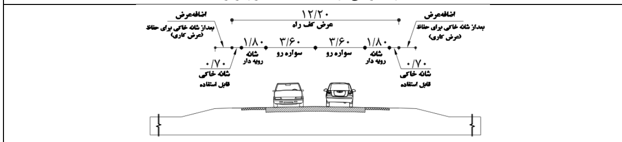
A4- راه شریانی دو خطه با ADT بیشتر از ۲۵۰
