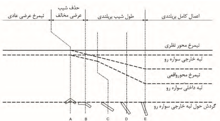
سواره رو با نیمرخ عادی حول لبه خارجی گردش می کند.
